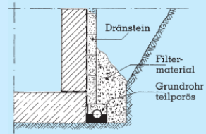
Dränstein und Grundrohr teilporös
