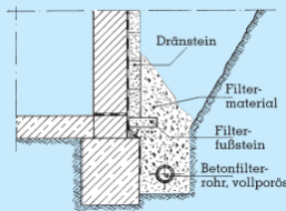
Dränstein, Filterfußstein und Betonfilterrohr vollporös
